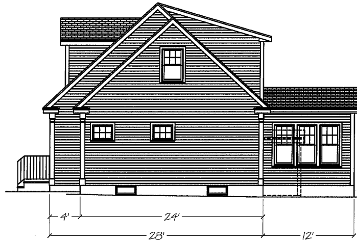
Right Elevation
