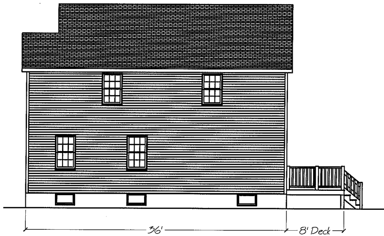
Right Elevation
