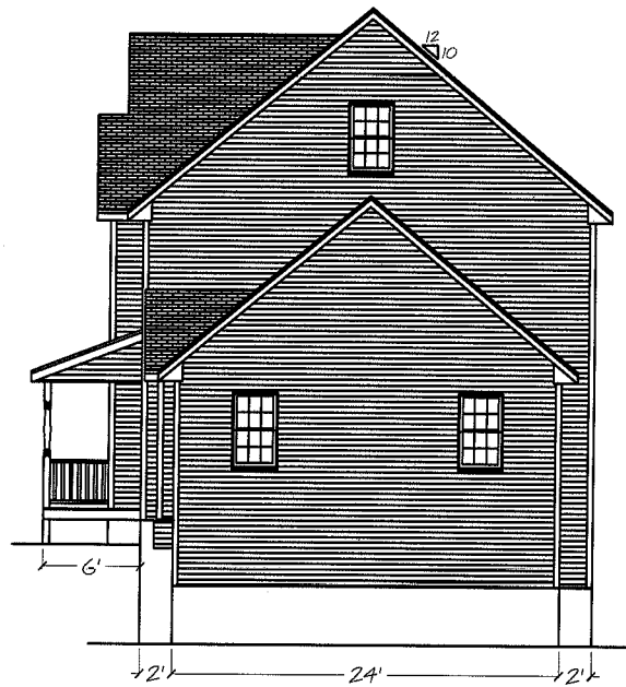
Right Elevation
