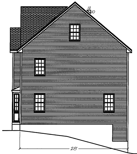
Right Elevation
