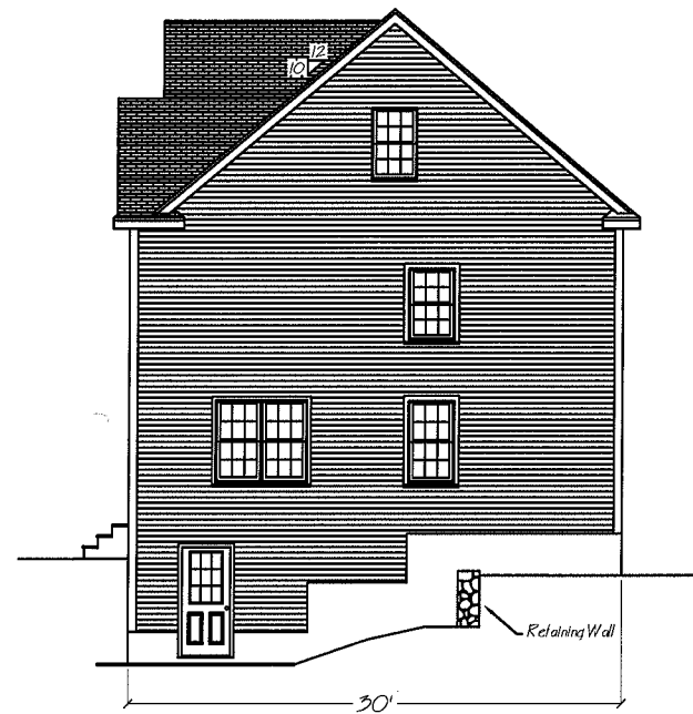
Right Elevation
