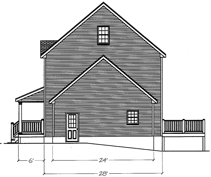
Right Elevation
