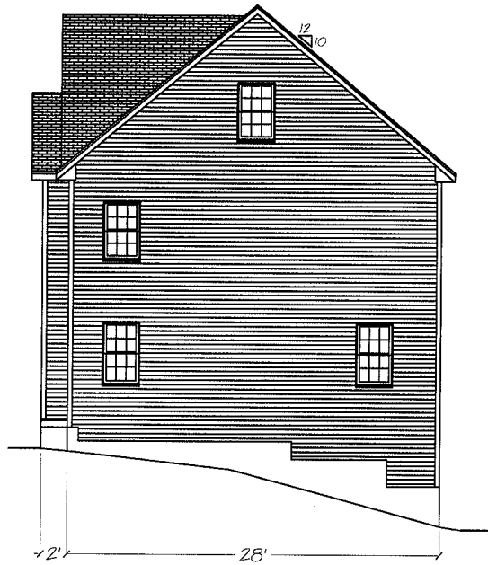
Right Elevation
