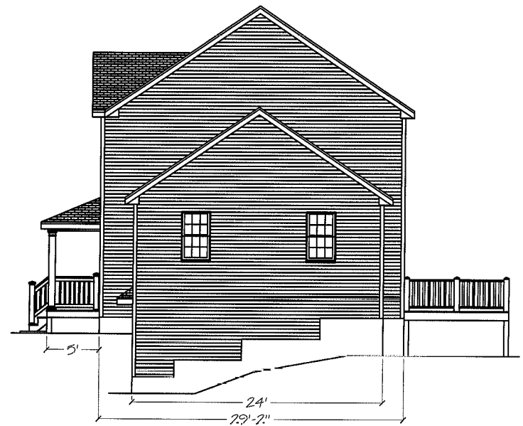
Right Elevation
