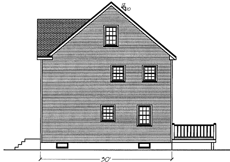
Right Elevation
