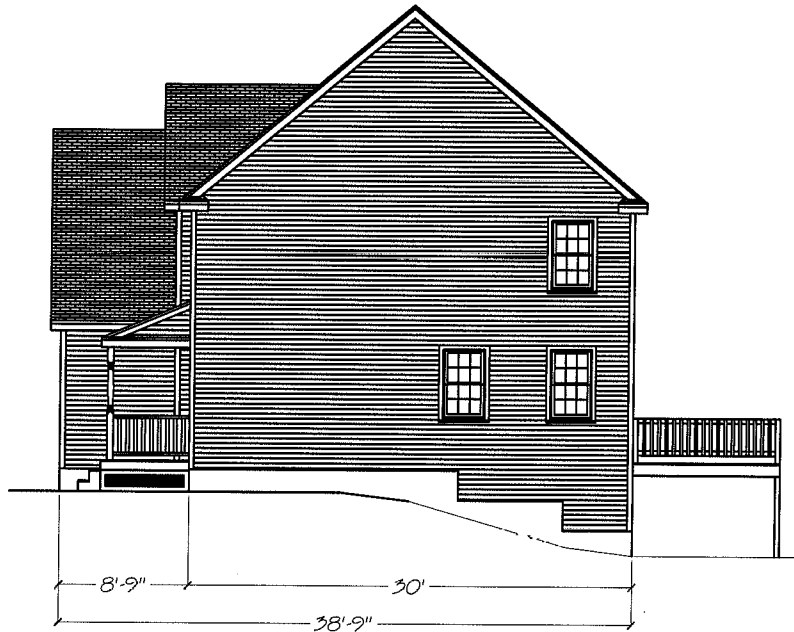
Right Elevation
