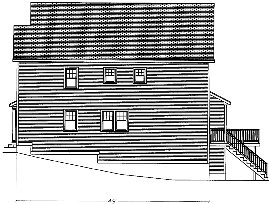
Right Elevation
