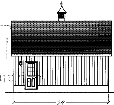
Right Elevation
