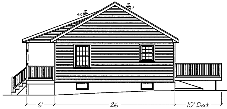
Right Elevation
