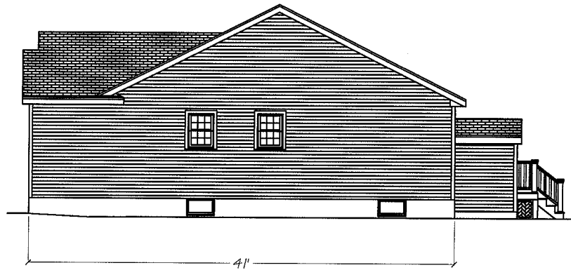
Right Elevation
